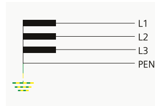
TN-C Sistem
